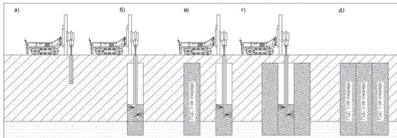
Технология стабилизации грунтов методом струйной цементации
