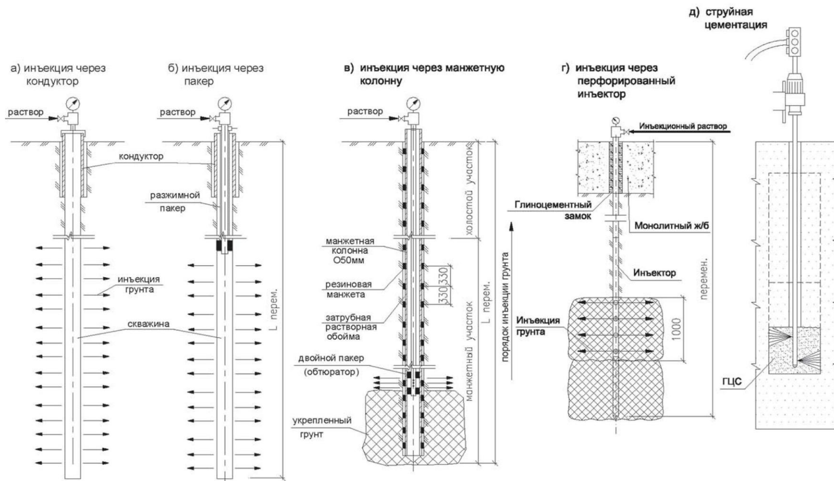
Рисунок В.1 – Оборудование скважин и способы инъекции
