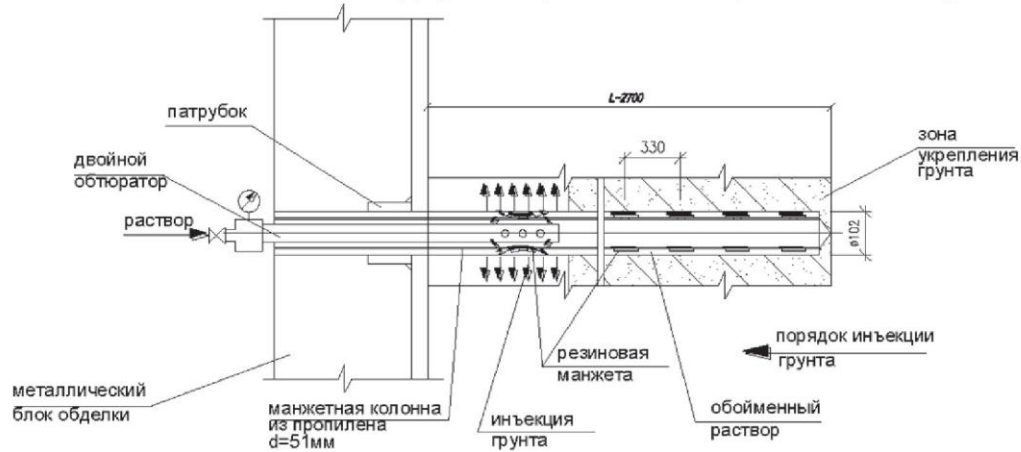
Рисунок Б.4 – Технологическая схема укрепления грунтов через манжетные колонны
