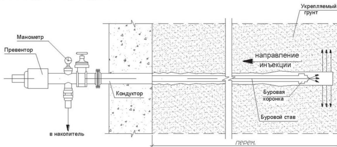
б) инъекция грунтов через буровой став
