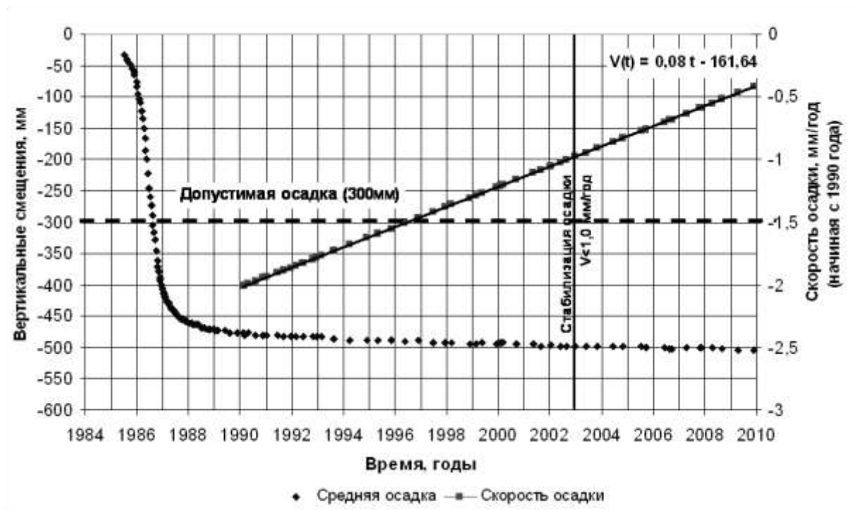
Рисунок Р.4 - График средних суммарных вертикальных смещений осадочных марок фундаментов
